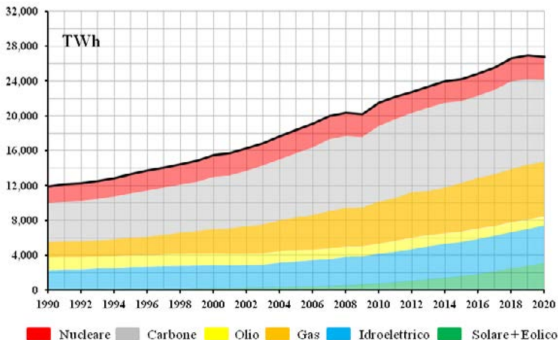
Figura 1. Produzione mondiale di energia elettrica negli ultimi 30 anni (TWh) e suddivisione nei contributi delle diverse fonti di energia
