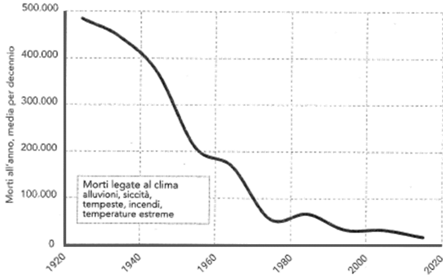
Fig. 4.4. Media per decennio delle vittime globali nei disastri legati al clima, tra il 1920 e il 2019.
