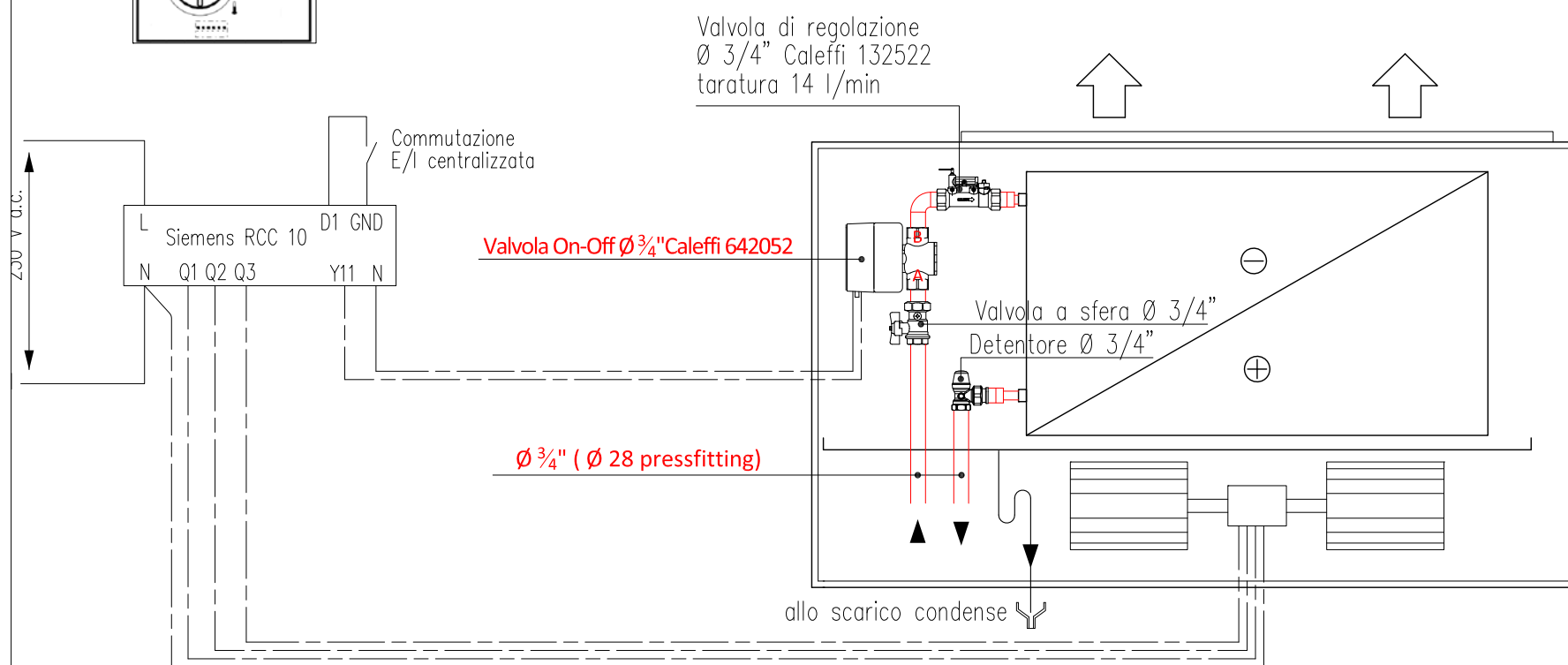
TIPICO INSTALLAZIONE VENTILCONVETTORE MASSIMA ALTEZZA DI POSA 2,80 m
