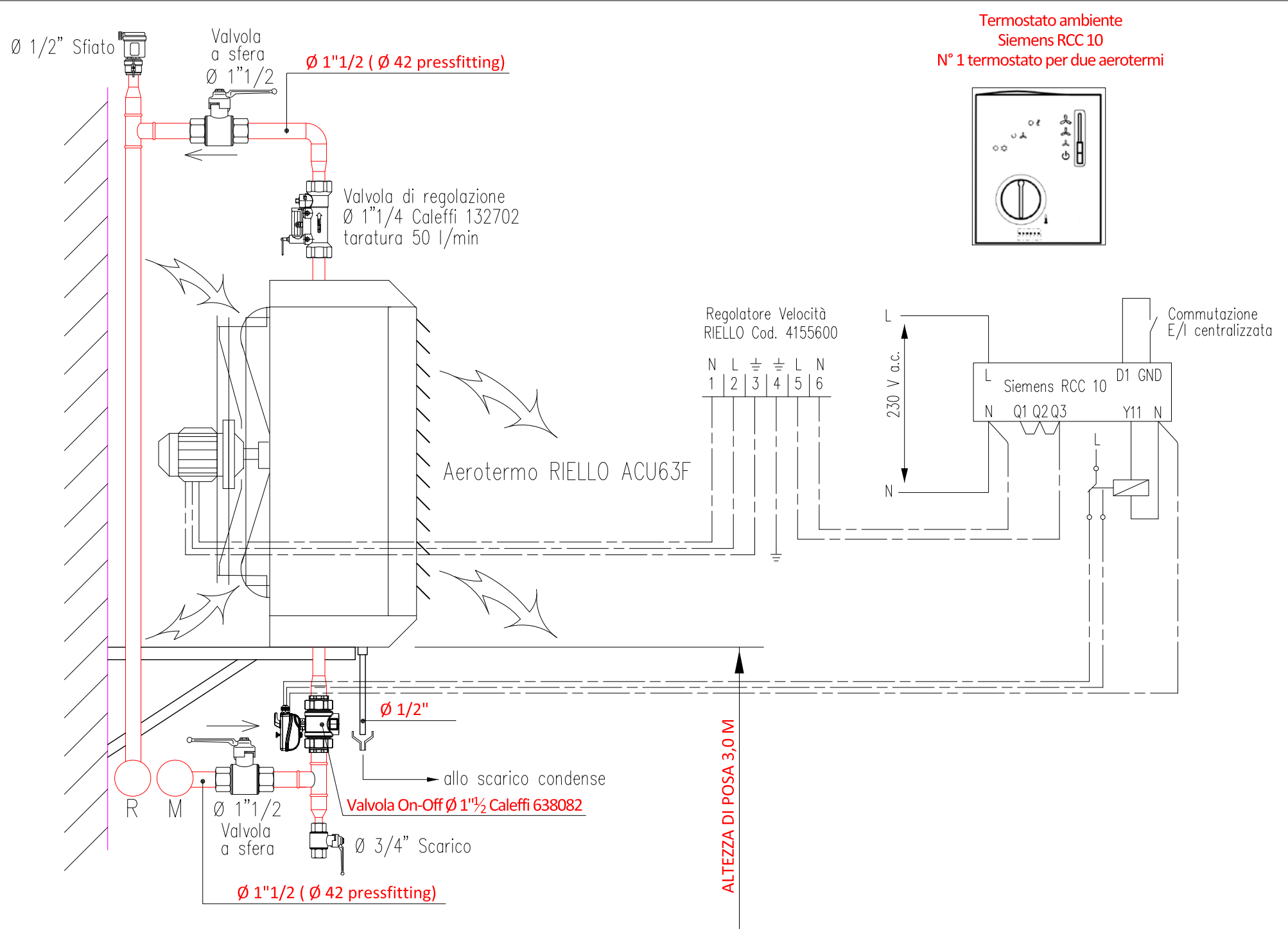
TIPICO INSTALLAZIONE AEROTERMO ALTEZZA ASSE DEL VENTILATORE 3,32 m
